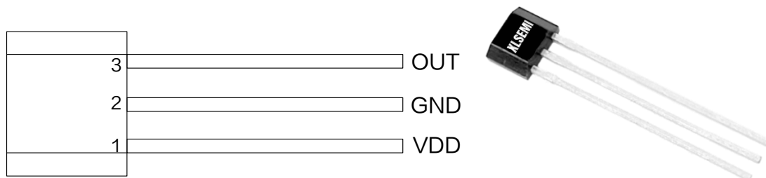
图 2. XL531 引脚配置
